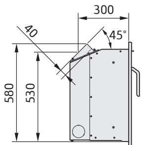
Rökrörsanslutning 45° bakåt
