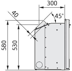
Rökrörsanslutning 45° bakåt
