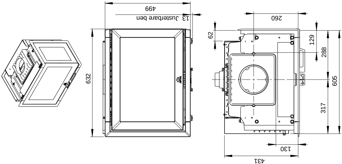
Jøtul I 520 FR
