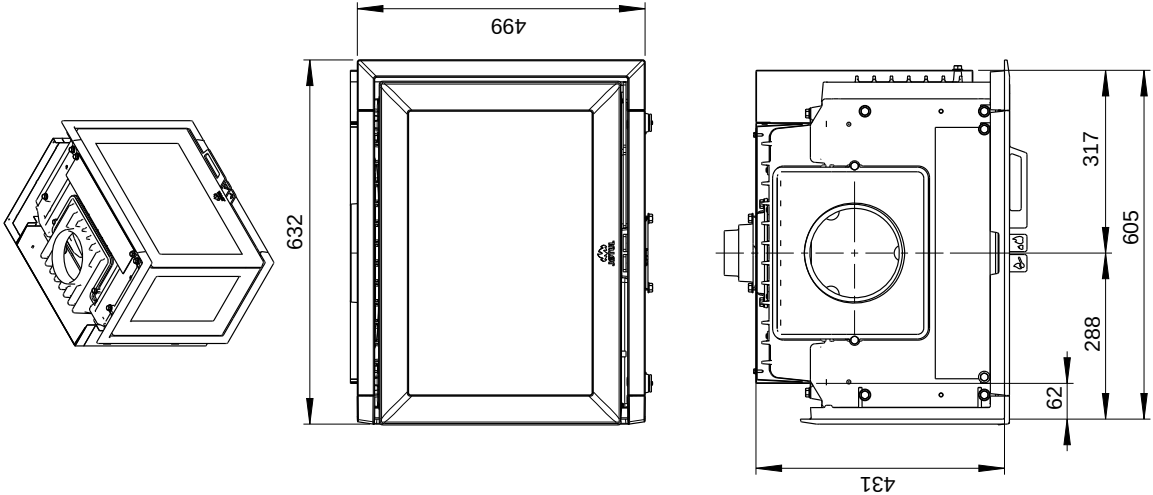
Jøtul I 520 FL
