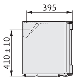
Rökrörsanslutning - Bakåt
