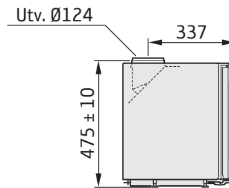
Rökrörsanslutning - Topp
